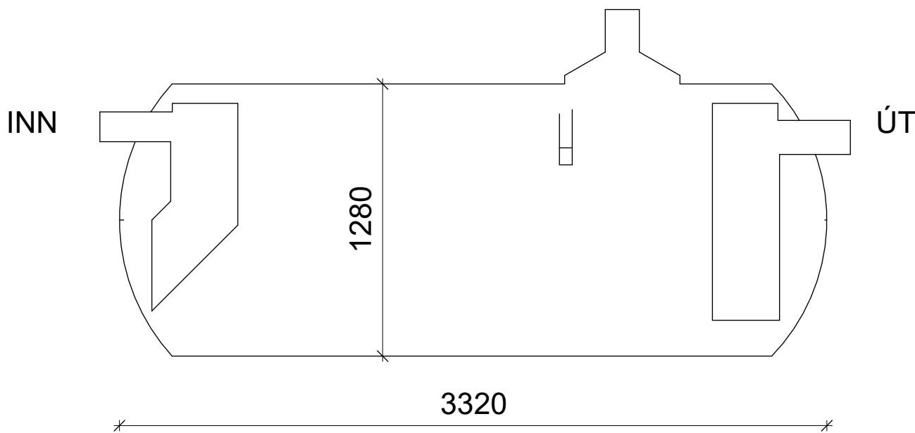
Fituskilja
